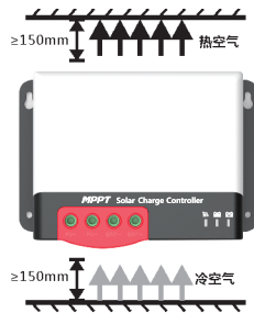
图2.1 安装和散热
