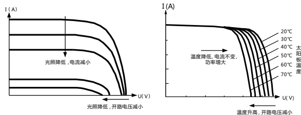
图1-3 电池板输出特性与光照的关系
