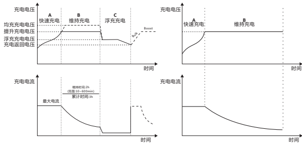
图1-5 铅酸电池充电阶段示意图
