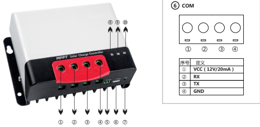
图1-1 控制器外观与接口
